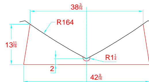
TRANSVERSAL SECTION "B" SECCION TRANSVERSAL "B"
